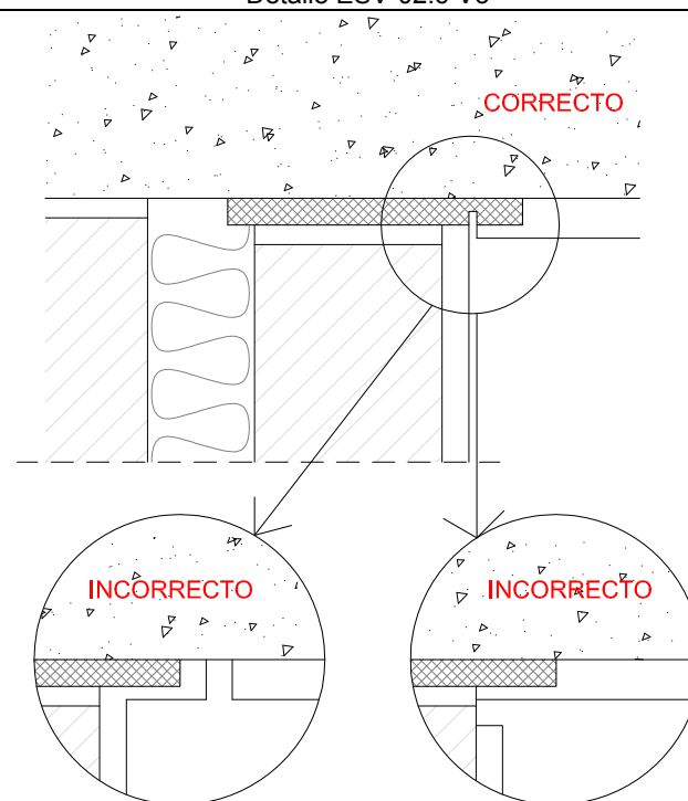
Detalle ESV-02.c-V6
