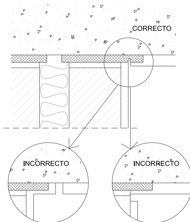
Detalle ESV-02.a.V4
