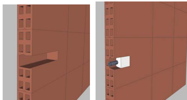
Detalle TAB-02.V2
