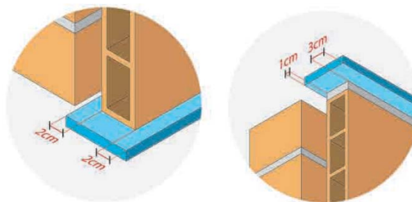
Detalle ESV-02.c-R4
