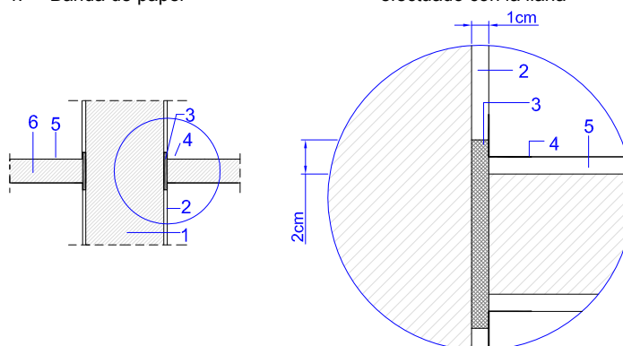
Detalle ESV-01.c.R2
