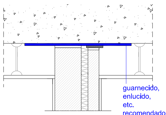
Detalle ESV-02.b-R8
