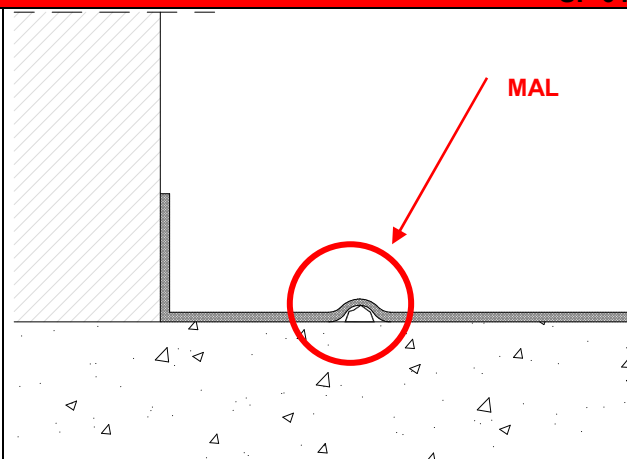
Detalle SF-01.b.V1
