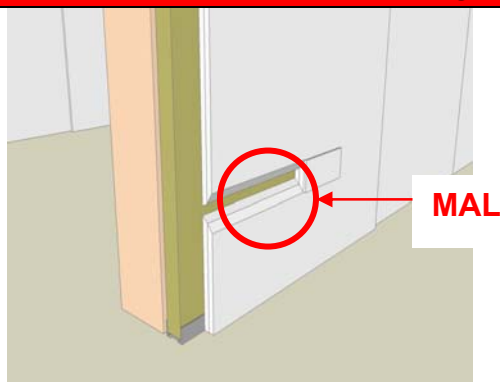
Detalle ESV-01.a.V3
