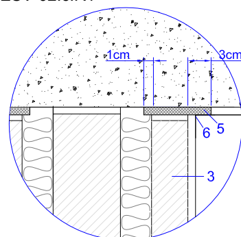
Detalle ESV-02.c.R2
