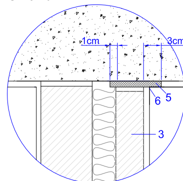
Detalle ESV-02.b.R2
