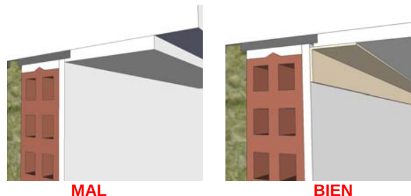
Detalle ESV-02.c-V5
