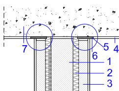
3. Detalle corte de la banda 4. Detalle tapado con cinta de papel. Detalle ESV-02.c.R1
