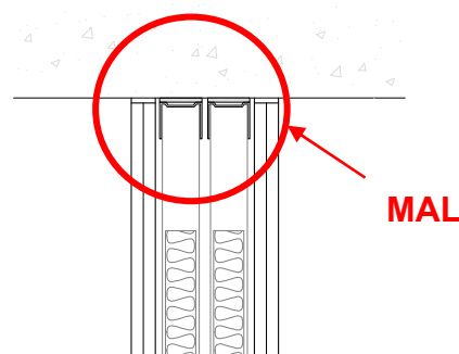
Detalle ESV-03.b.V2
