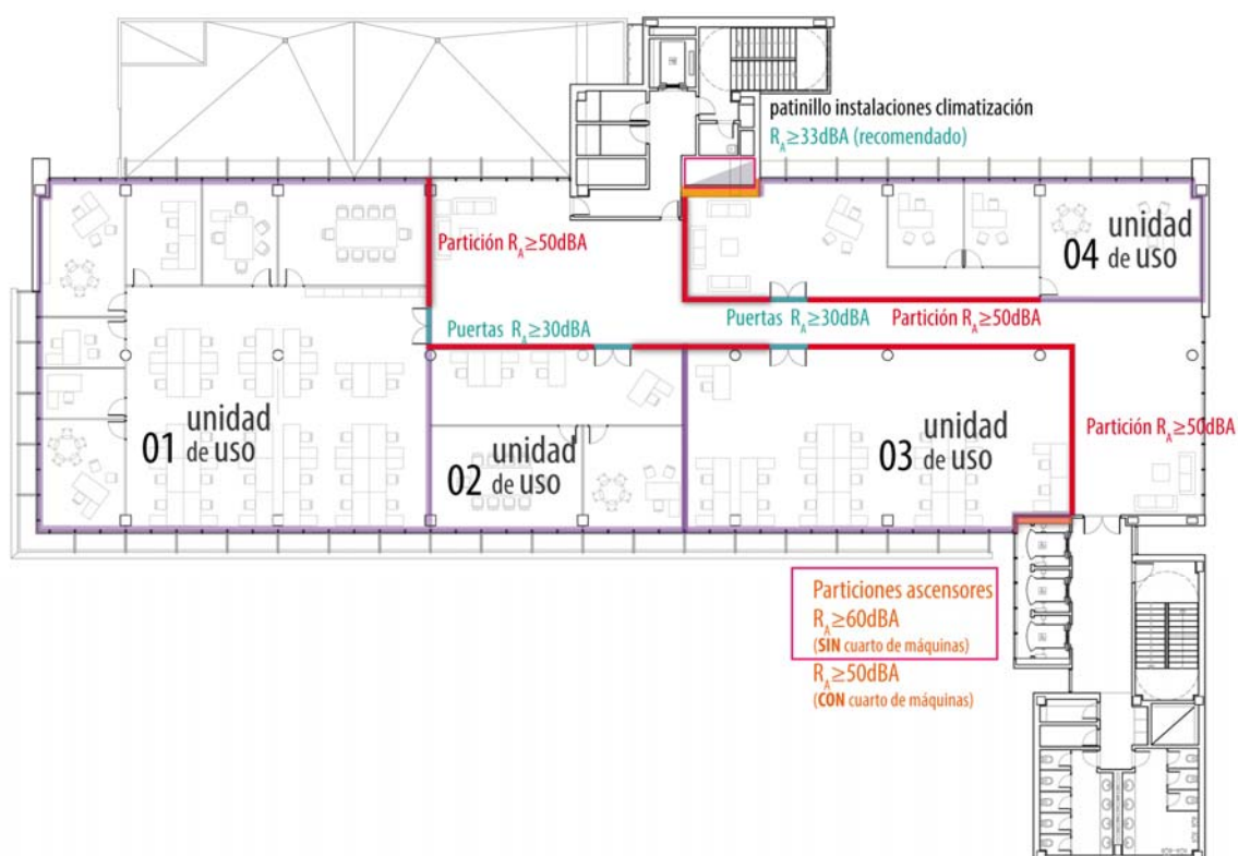
Figura A2.54. Planta tipo del edificio y valores de aislamiento acústico a ruido aéreo exigidos a los elementos constructivos con puertas, los ascensores y los conductos de ventilación
