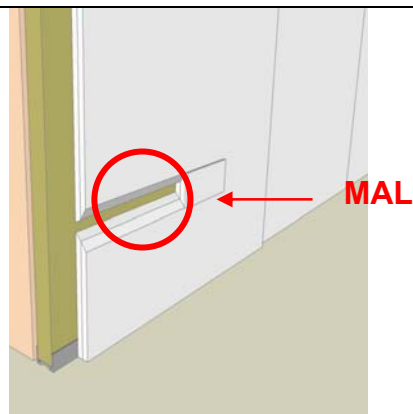
Detalle ESV-03.b.V4
