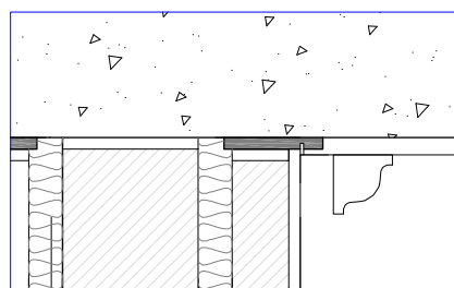
Detalle ESV-02.c-R6
