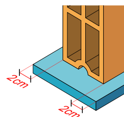
Detalle ESV-02.b-R4
