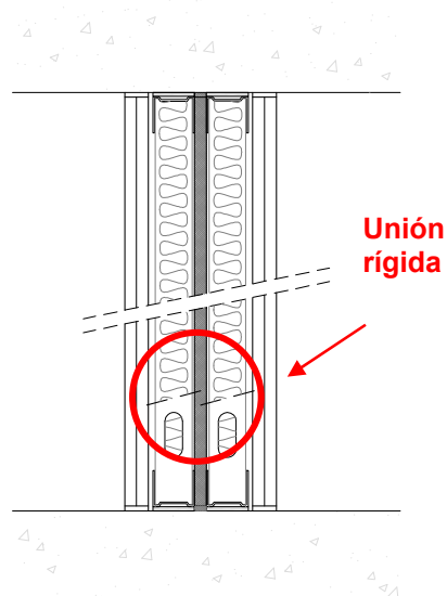
Detalle ESV-03.a.V1
