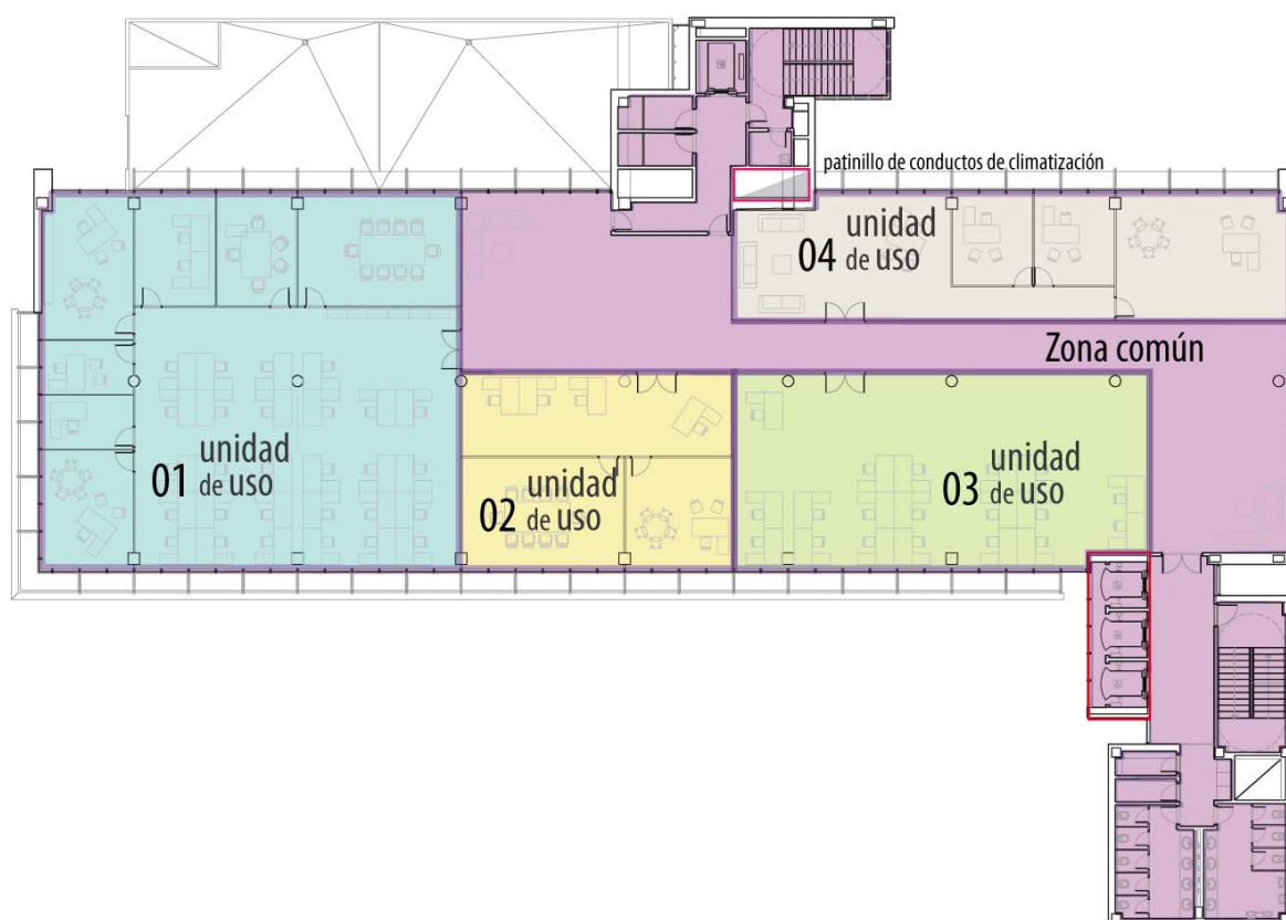
Figura A2.51. Zonificación de la planta tipo
