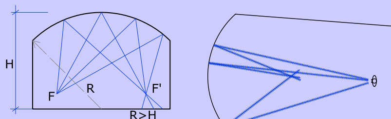
Figura 2.2.2. Vista en sección (izquierda) y en planta (derecha) de aulas con paramentos curvos donde se dan concentraciones en determinados puntos del recinto.
