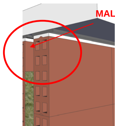
Detalle ESV-02.c-V2
