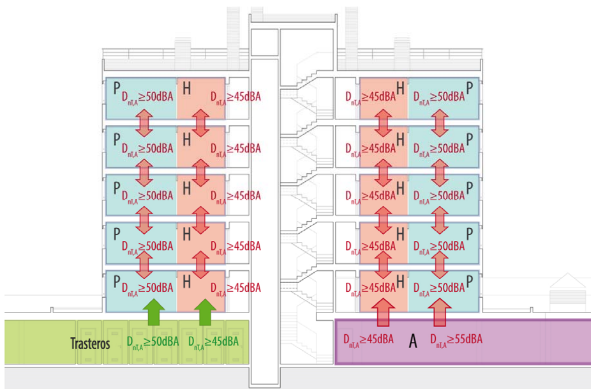
Figura A2.5. Valores de aislamiento acústico a ruido aéreo exigidos. Sección
