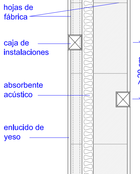
PLANTA Detalle ESV-02.b-R7
