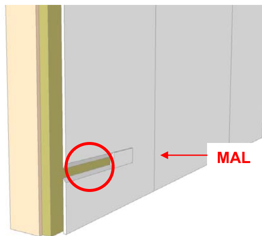
Detalle ESV-01.b.V1
