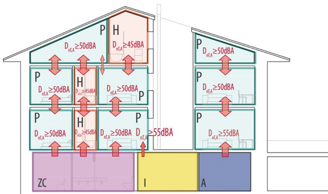
Figura A2.18. Valores de aislamiento acústico a ruido aéreo exigidos. Sección 02 transversal por cuarto de instalaciones
