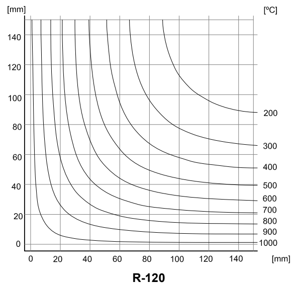
Figura C.6. Isotermas para cuartos de sección de 300 x 300 mm expuestos por ambas caras
